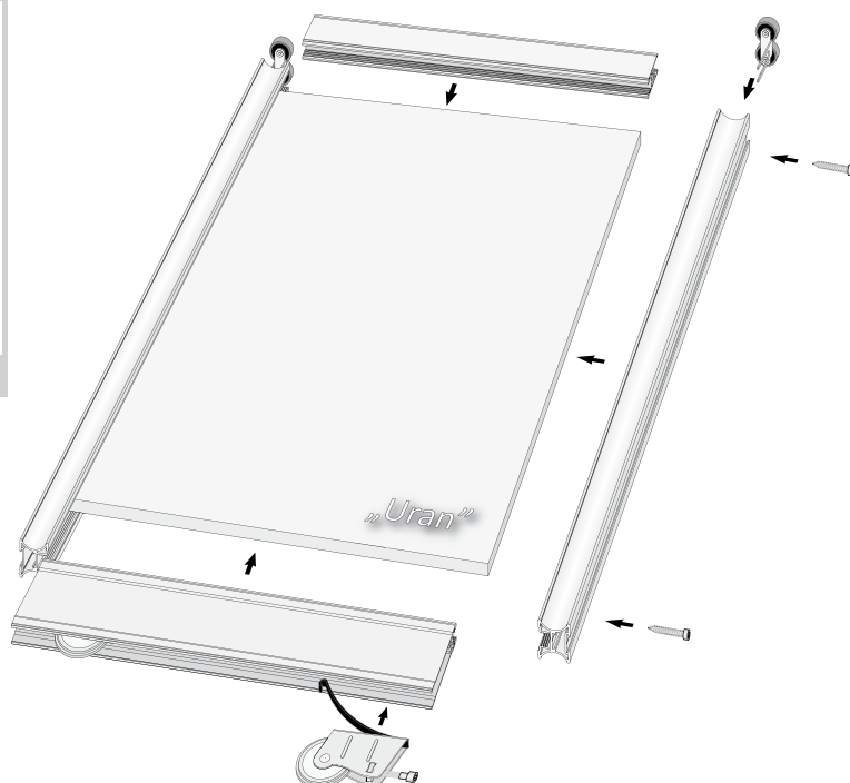
Montáž kolejnic
